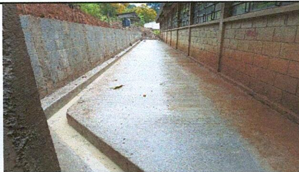
Foto 5: TERMINACIÓN DE MURO DE CONTENCIÓN CON DRENAJE FRANCES
