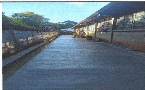
Foto2: TERMINACIÓN LOSA DE PISO MURO DE CONTENCIÓN CON DRENAJE FRANCES
