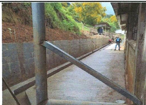
Foto 4: TERMINACIÓN DE DE LOSA DE PISO
